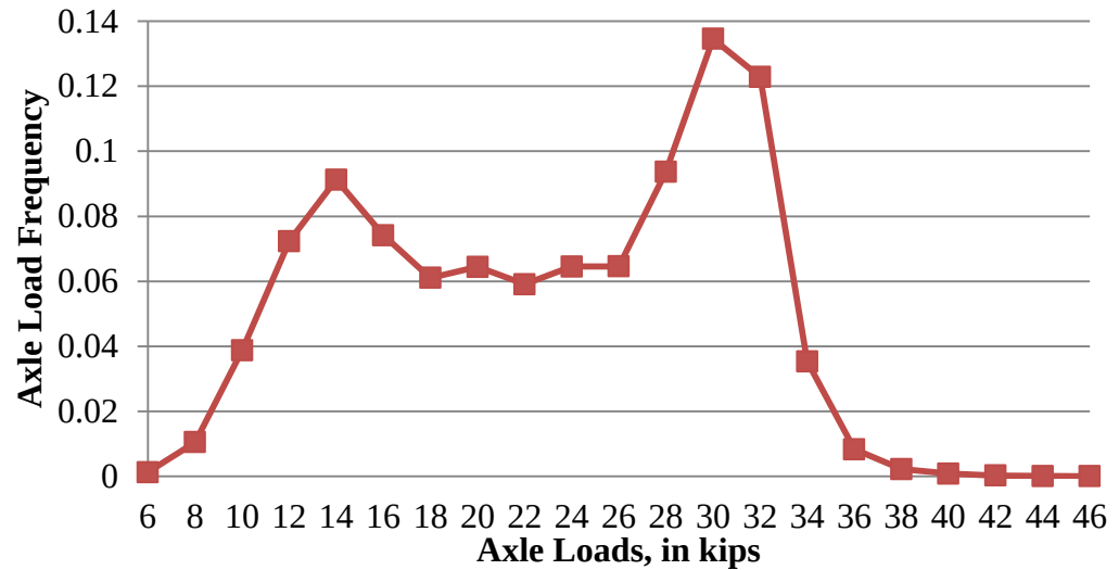
FIGURE 1.2 The tandem ALS of WIM Station 961 in August 2007
